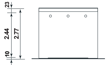
Rückansicht
