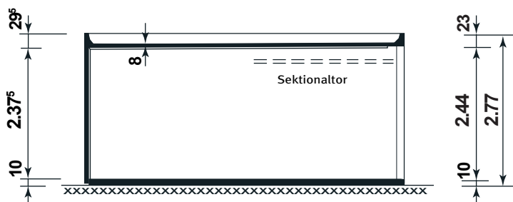
Schnitt
