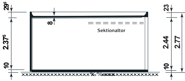
Schnitt
