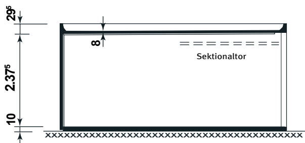
Schnitt
