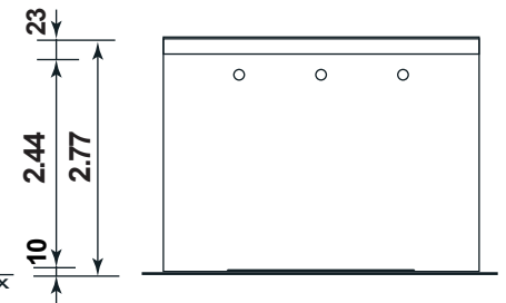
Rückansicht
