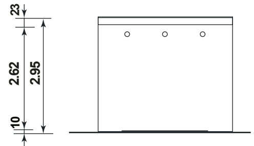
Rückansicht
