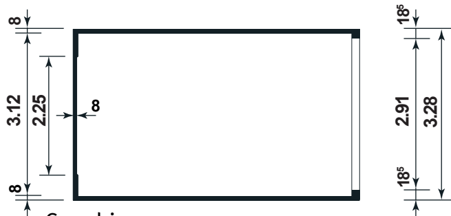
Grundriss
