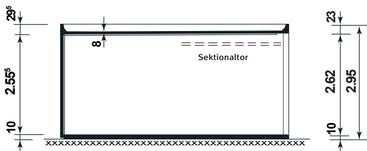
Schnitt
