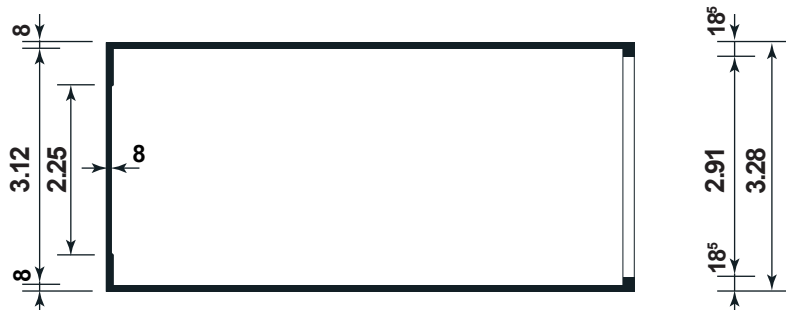
Grundriss
