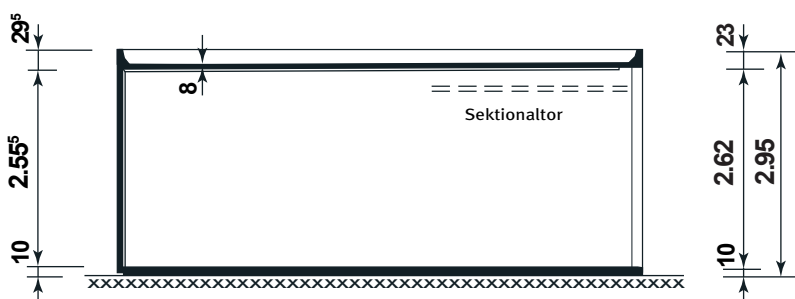
Schnitt
