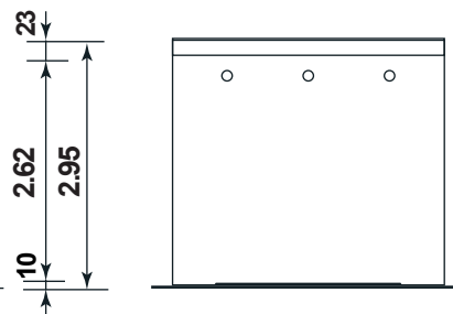
Rückansicht
