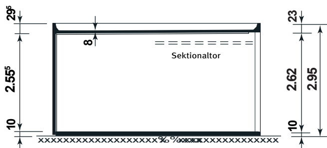
Schnitt
