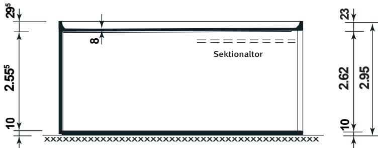
Schnitt
