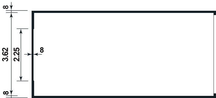
Grundriss
