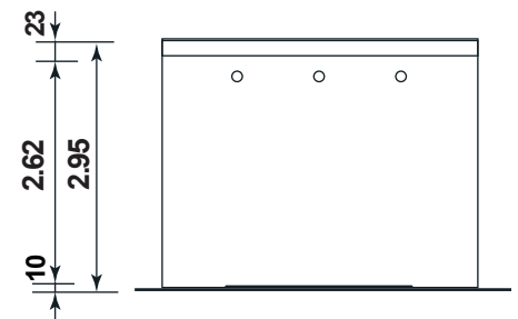
Rückansicht
