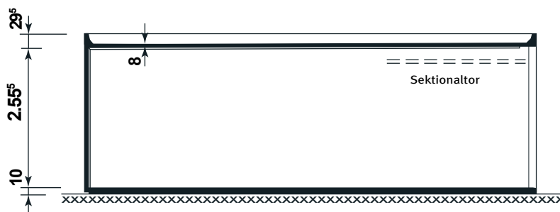
Schnitt
