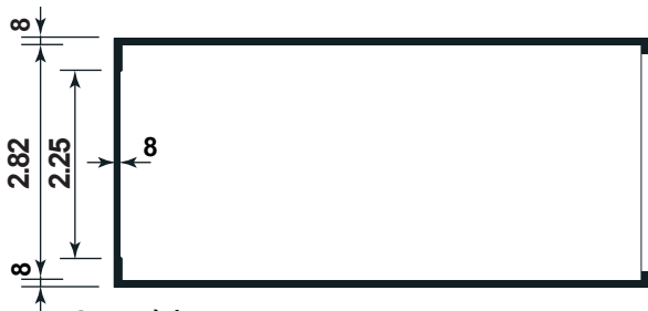
Grundriss
