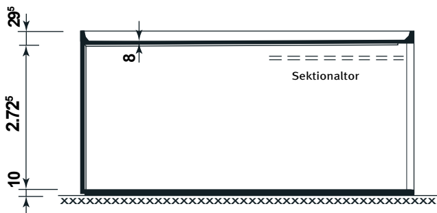
Schnitt
