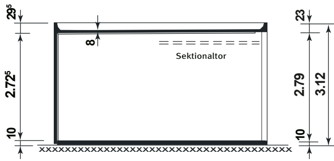
Schnitt
