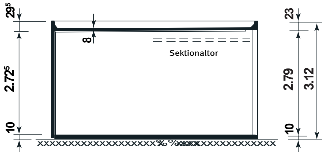
Schnitt
