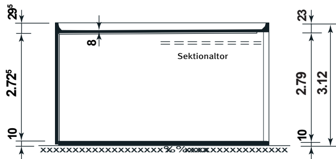
Schnitt
