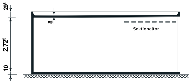
Schnitt
