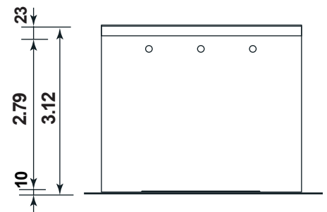
Rückansicht
