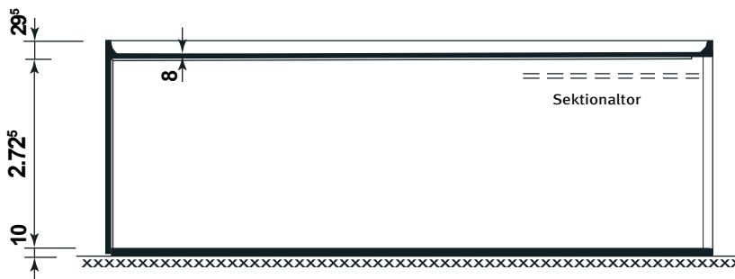
Schnitt
