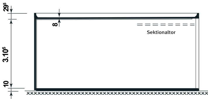
Schnitt
