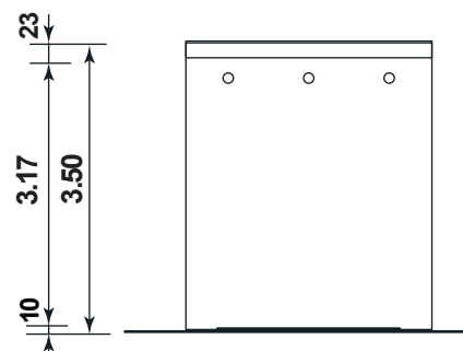
Rückansicht
