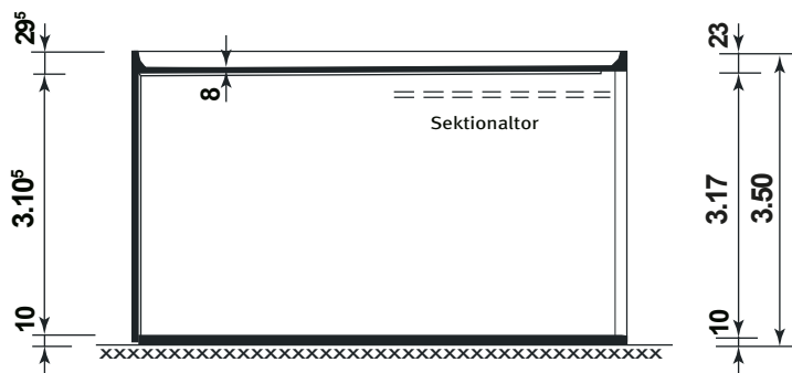
Schnitt
