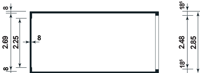
Grundriss
