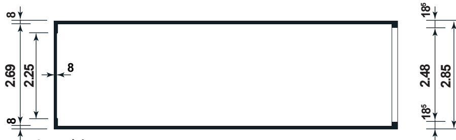
Grundriss
