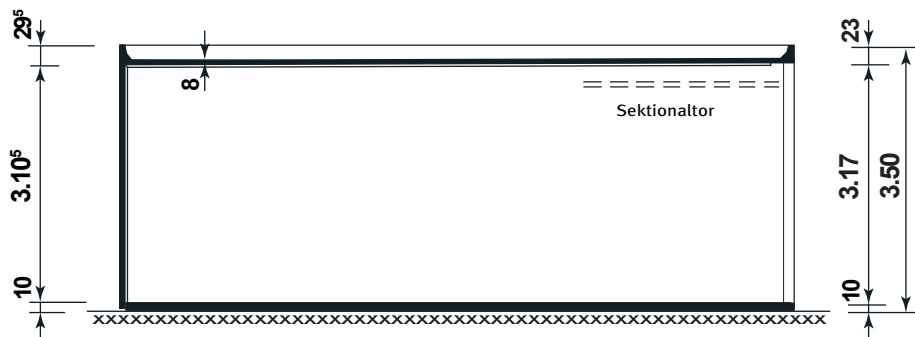
Schnitt
