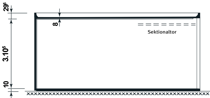
Schnitt
