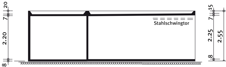
Schnitt
