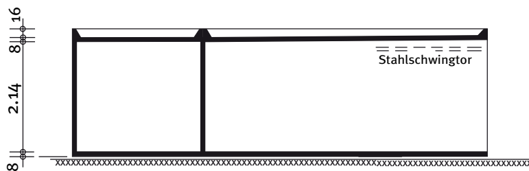
Schnitt
